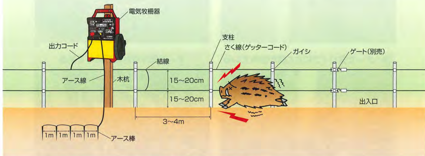
イノシシ用セットの設置概要図
