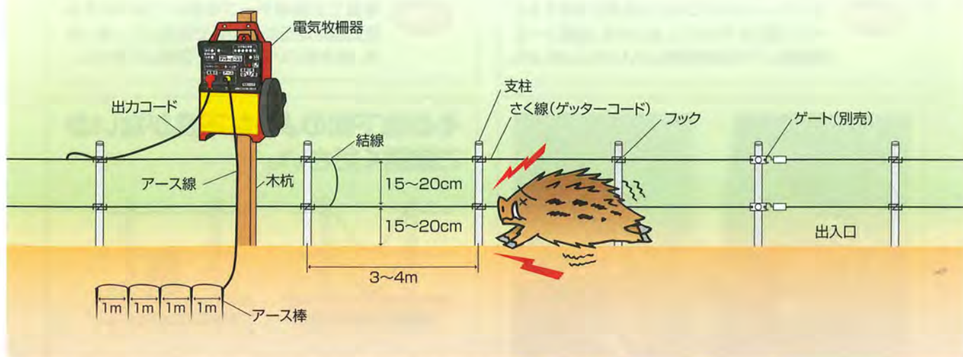
イノシシ用FRPセットの設置概要図
